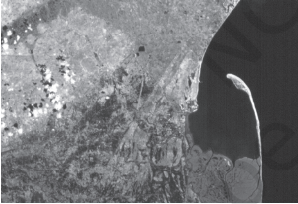
चित्र 7.14 : उपग्रहीय चित्र-गोदावरी नदी डेल्टा का स्पिट
