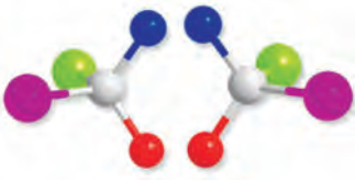
चित्र 10.7- एक काइरल अणु एवं उसका दरपण प्रतिबिंब
