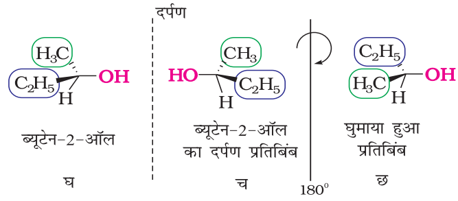
चित्र 10.6- 'घ' के प्रतिबिंब रूप 'च' को 180° घुमाने पर 'छ' प्राप्त होता है 'छ' को 'घ' पर अध्यारोपित नहीं कर सकते।
