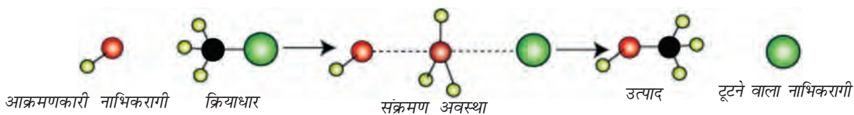
चित्र 10.2- लाल गेंद आक्रमणकारी हाइड्रॉक्साइड आयन को तथा हरी गेंद निकलने वाले हैलाइड आयन को प्रदर्शित करती है।
