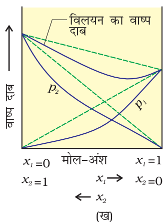
चित्र 2.6— द्विघटकীয় निकाय का वाष्प दाब उनके संघटन के कारक के रूप में (क) राउल्ट के नियम से धनात्मक विचलन दर्शाने वाला विलयन (ख) राउल्ट के नियम से ऋणात्मक विचलन दर्शाने वाला विलयन
