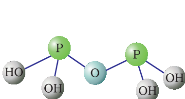
(H_4P_2O_7) पायरोफॉस्फोरस
