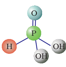
H_3PO_3 आर्थोफॉस्फोरस अम्ल
