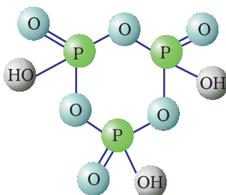
(HPO_3)_3 साइक्लोट्राइमेटाफॉस्फोरिक अम्ल
