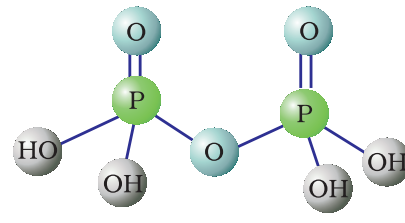
H_4P_2O_7 पायरोफॉस्फोरिक अम्ल
