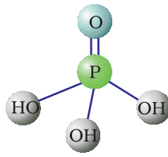
H_3PO_4 आर्थोफॉस्फोरिक अम्ल
