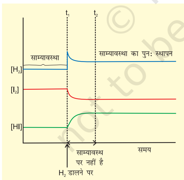
चित्र 7.8 H_2(g) + I_2(g) \rightleftharpoons 2HI(g) अभिक्रिया में साम्यावस्था पर H_2 के डालने पर अभिकारकों एवं उत्पादों के सांद्रण में परिवर्तन
